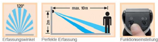
Erfassungswinkel 120°
